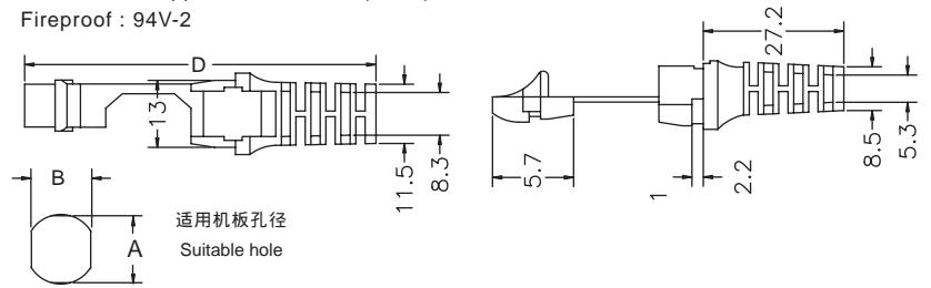
单位/Unit:mm
